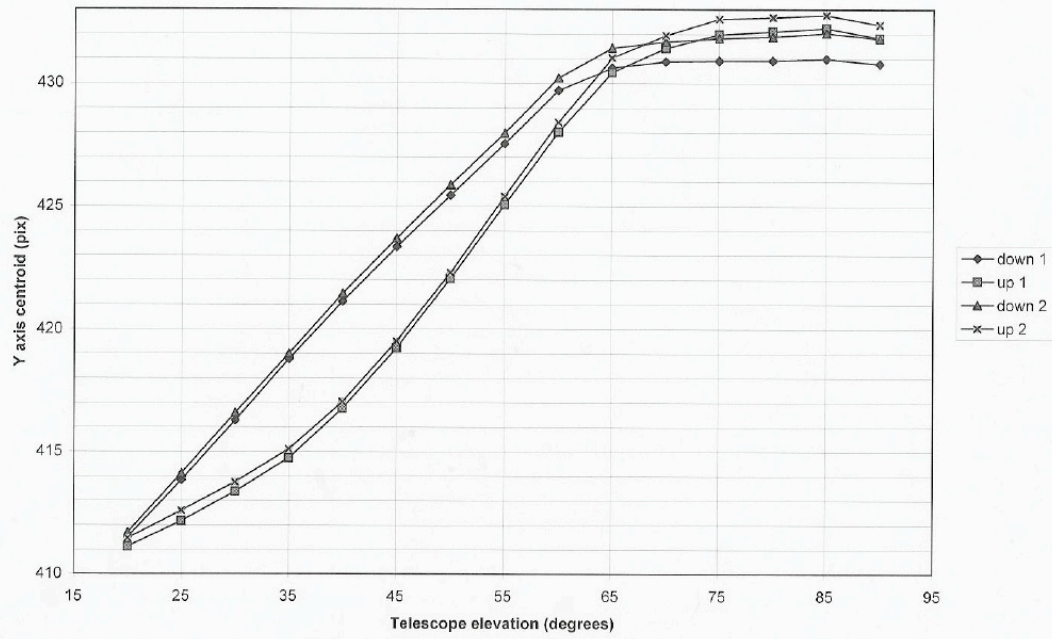
Y Axis Flexure
