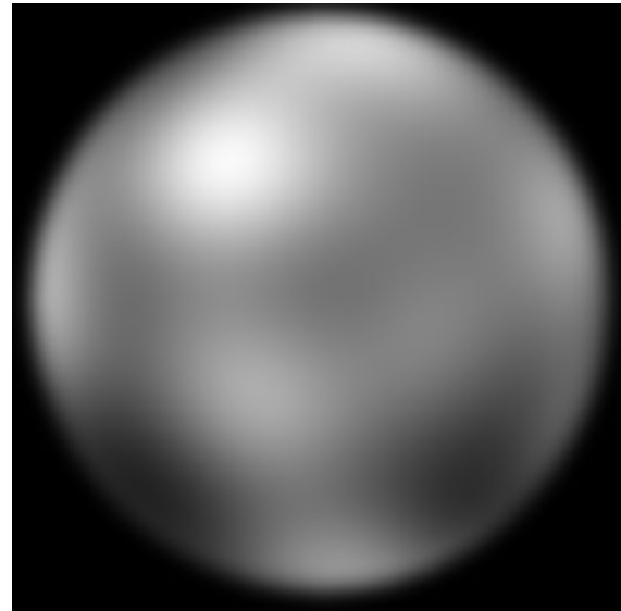
Pluto
