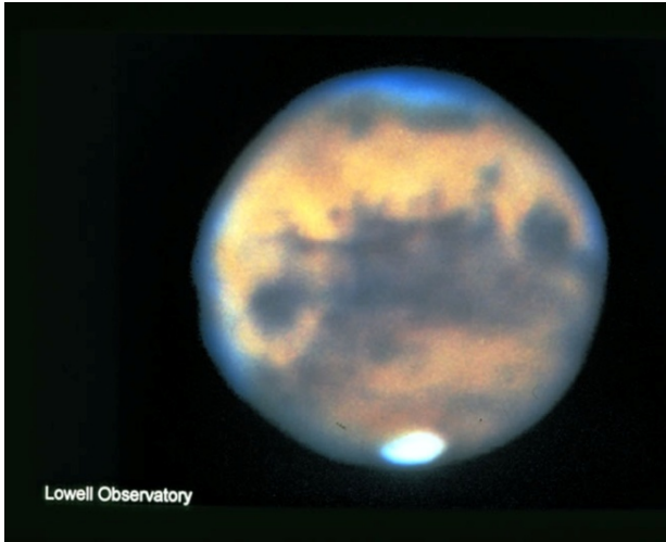
Mars
