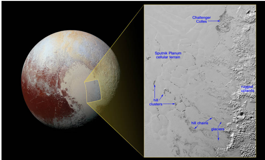
Pluto
