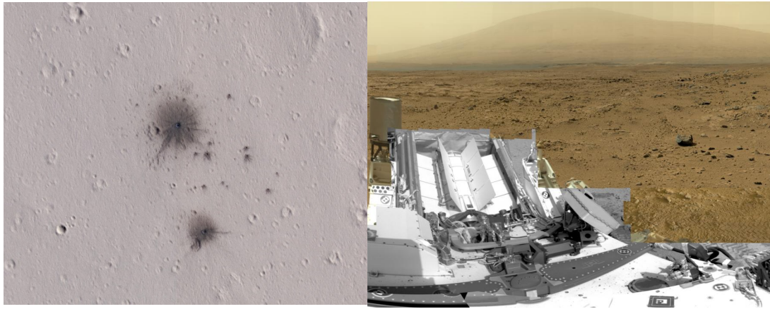
Mars
